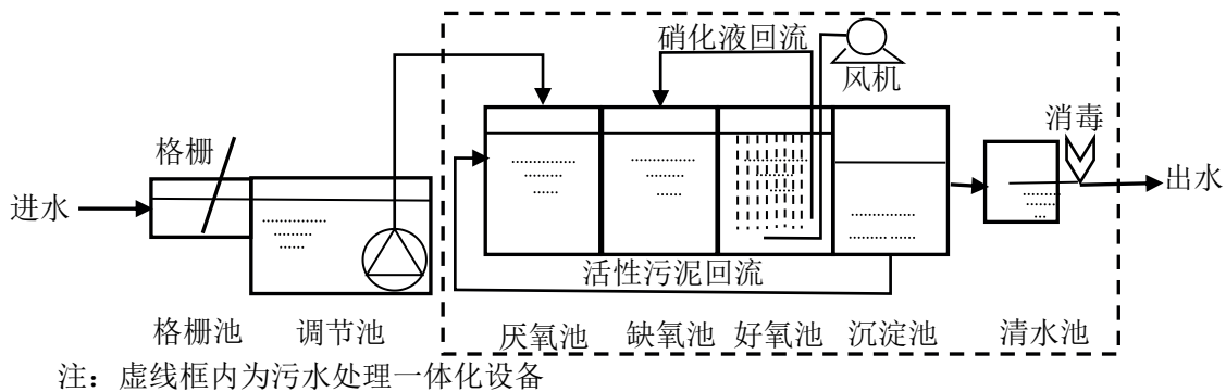
图 2 A 2 /O 污水处理工艺流程图
