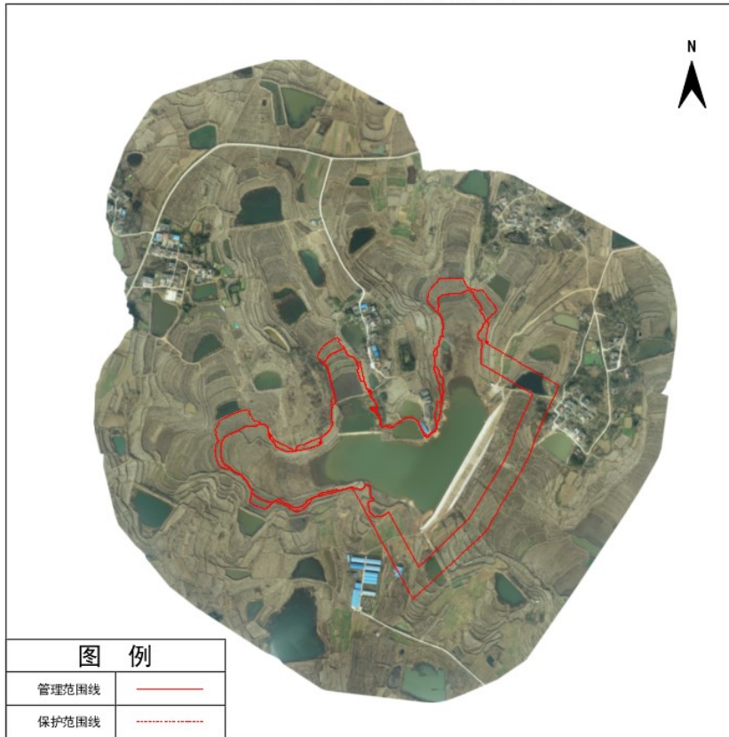
光山县石庄水库管理与保护范围线公示图
