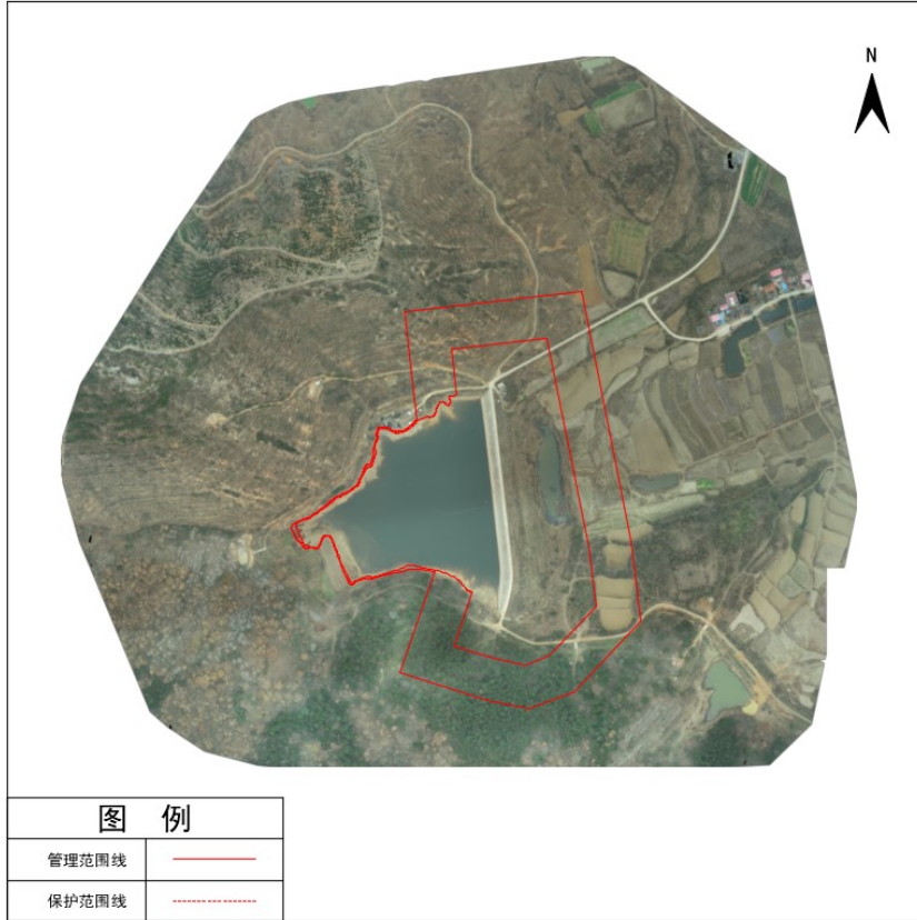
光山县河洼水库管理与保护范围线公示图
