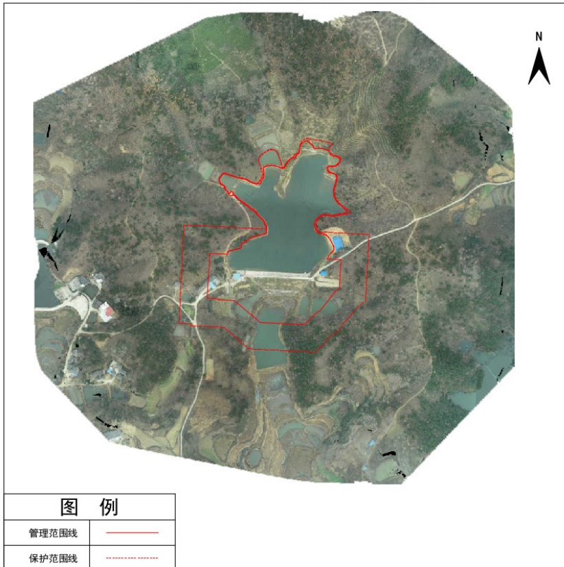
光山县上庄水库管理与保护范围线公示图
