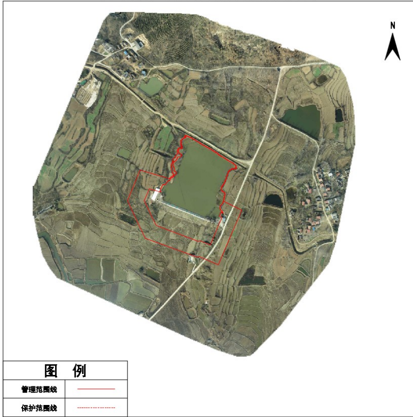
光山县肖咀水库管理与保护范围线公示图
