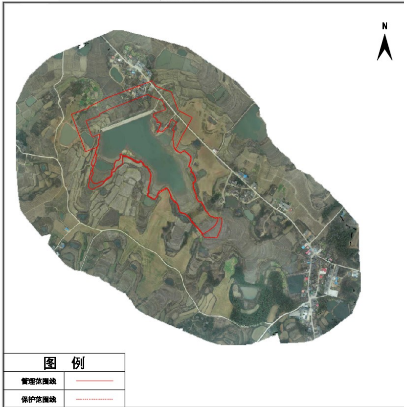
光山县高涂湾水库管理与保护范围线公示图
