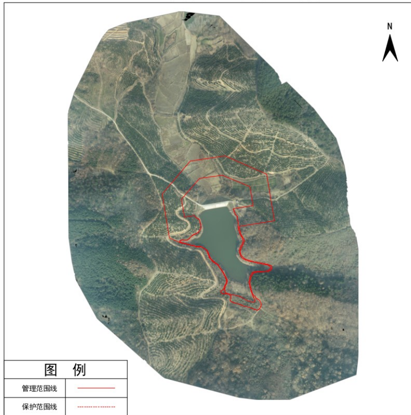
光山县柳木洼水库管理与保护范围线公示图
